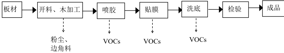
图 2-1 吸塑门板生产工艺流程图
