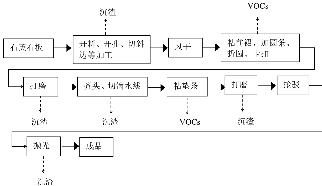
图 2-3 石英石台面生产工艺流程图
