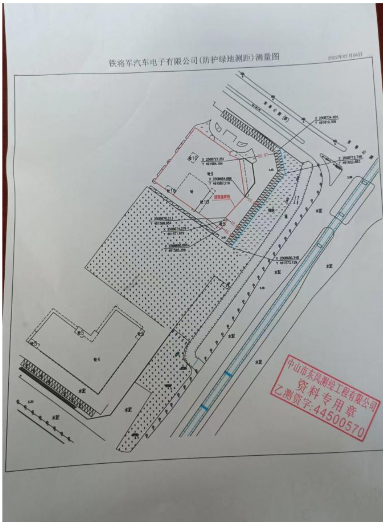
附件 2 防护绿地测距 (测量图)
