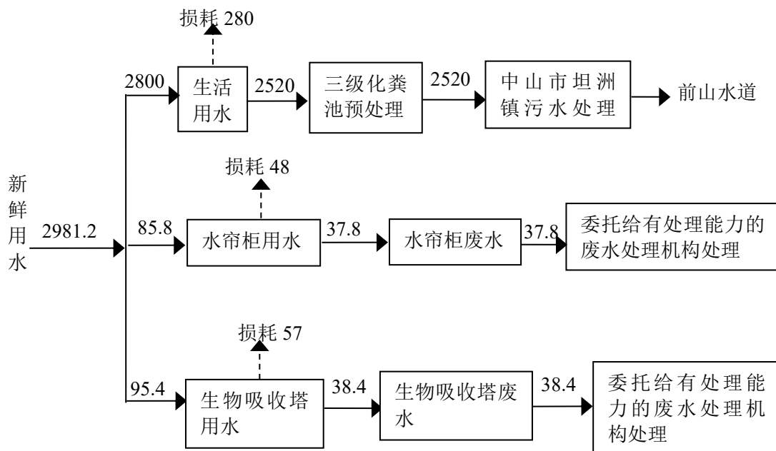
图 1 项目迁建后水平衡图 (t/a)
