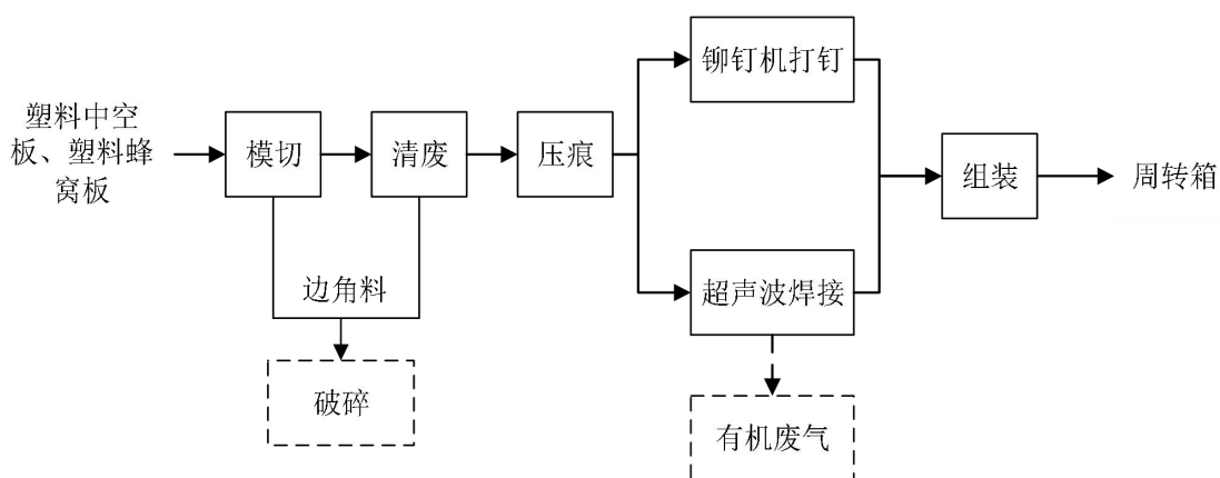
图3 周转箱生产工艺流程图
