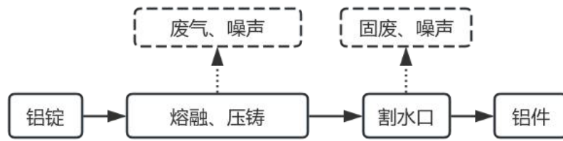
图3 改扩建前铝件生产工艺流程图
