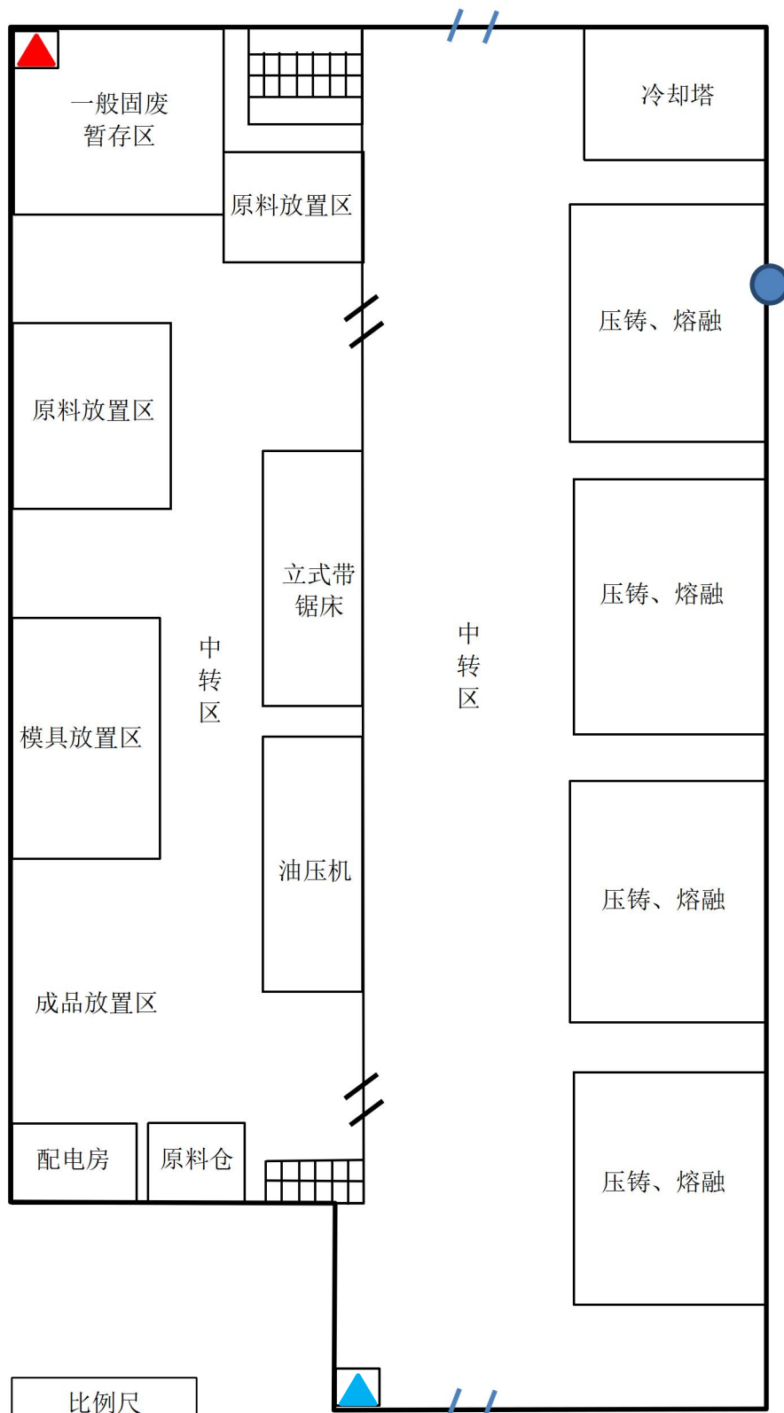
附图 3 车间平面布置图
