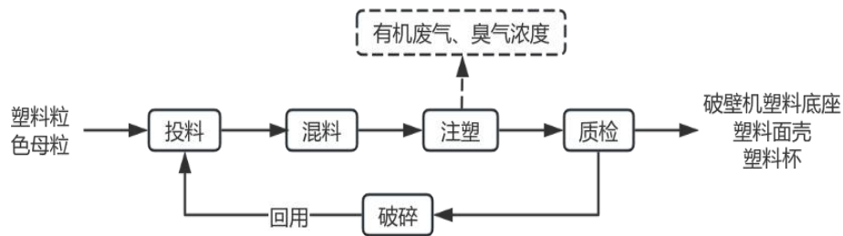
图2 破壁机塑料底座、塑料面壳、塑料杯生产工艺流程图
