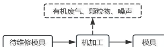
图5 模具维修工艺流程图
