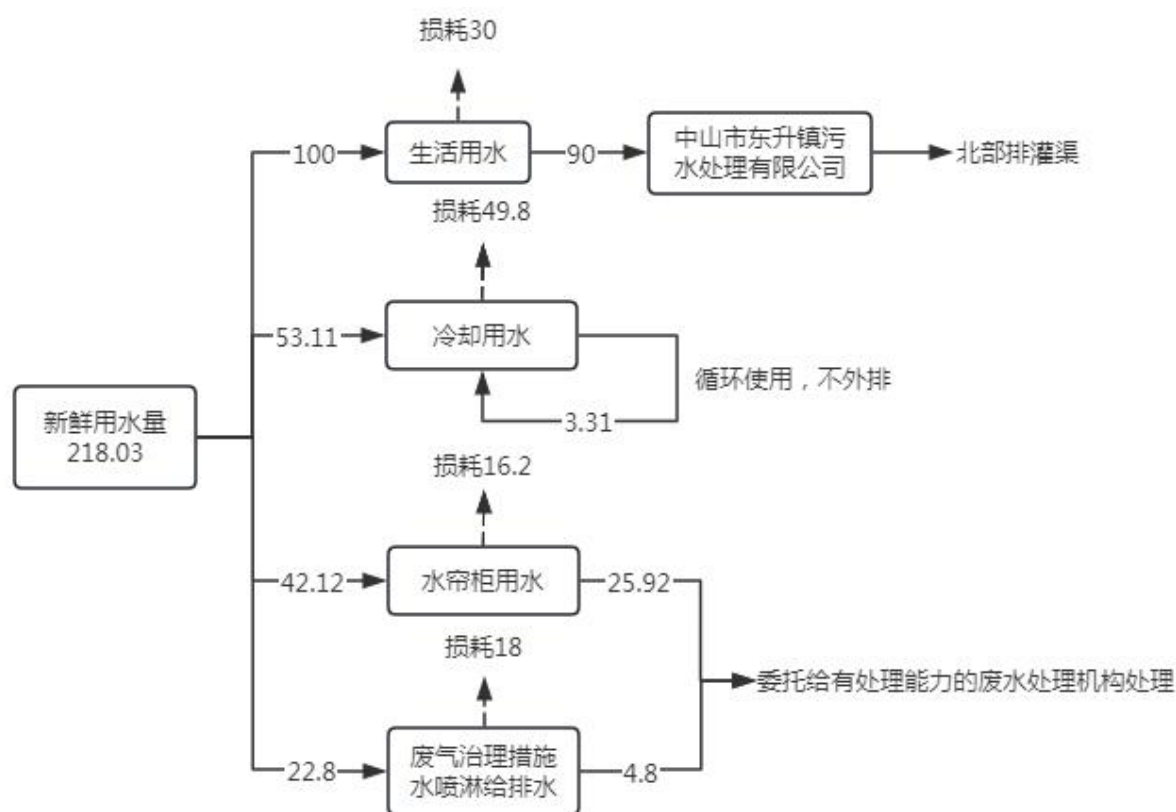
图 1 项目实际水平衡图（单位：t/a）
