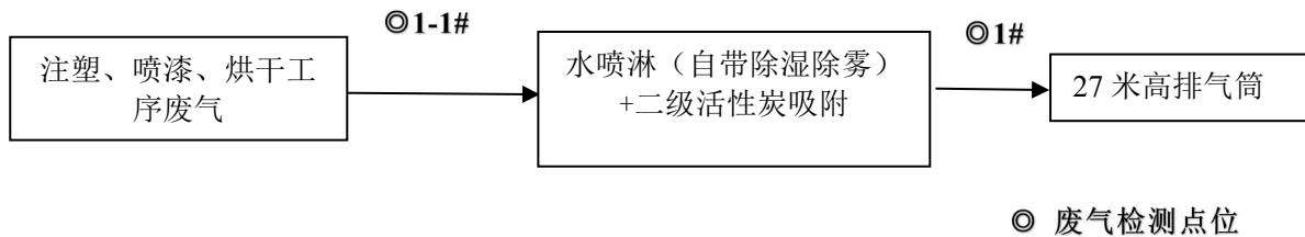
图 3-1 废气处理工艺流程图
