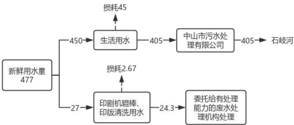
图 1 项目水平衡图 t/a
