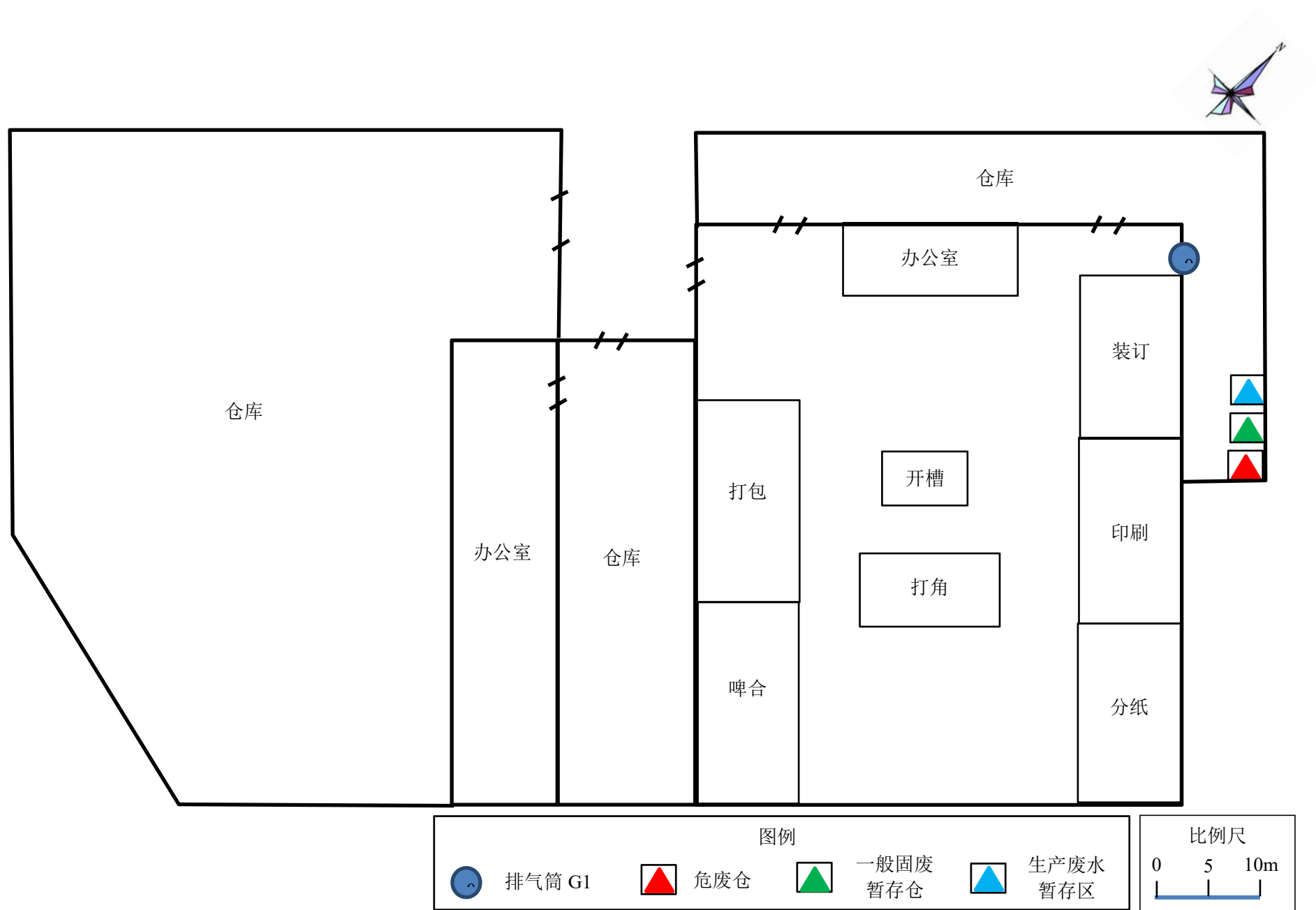
附图 3 建设项目平面布置图
