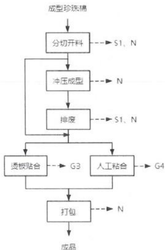
图2-2 珍珠棉包装制品生产工艺流程图
